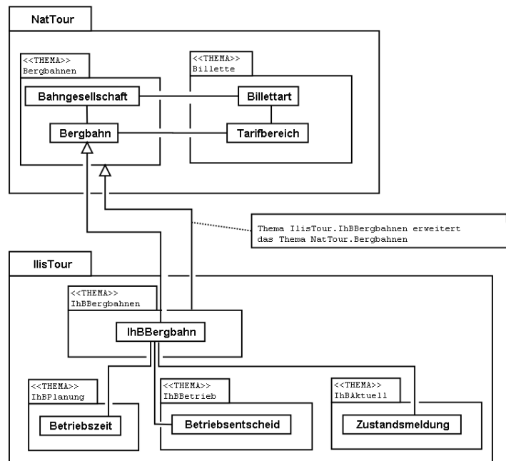
Abbildung 15: Das Ilistaler Modell (IIsTour) erweitert das Modell des nationalen Tourismus-Verbands (NatTour). IIsTour erbt das Thema Bergbahnen von NatTour, erweitert die Klasse Bergbahn zu IhBBergbahn und fügt weitere Themen für Planung, Betrieb und Aktuelles an.
