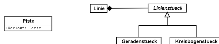
Abbildung 39: Der Verlauf einer Piste ist eine Linie. Diese bestehen ihrerseits aus einzelnen Linienstücken, von denen es verschiedene Arten gibt: Geradenstücke, Kreisbogenstücke, etc.
