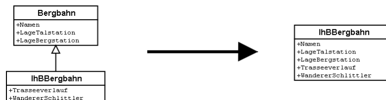
Abbildung 17: Das Programmpaket für den Ilistaler Tourismus braucht sich nur grob ans konzeptuelle Modell zu halten. Es kann zum Beispiel intern zwei Objektklassen zu einer einzigen zusammenfassen. Wichtig ist nur, dass das Paket in der Lage ist, die Daten in jenem Format zu liefern, das dem konzeptuellen Modell entspricht.
