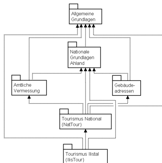
Abbildung 12: Das Ilistaler Tourismus-Datenmodell (IlistTour) braucht nicht alles selbst zu definieren. Stattdessen baut es auf anderen Modellen auf: Es verwendet Teile des nationalen Tourismus-Modells (NatTour), der nationalen Grundlagen von Ahland, der amtlichen Vermessung, der Gebäudeadressen sowie allgemeine Grundlagen. Die gestrichelte Linie mit gefülltem Pfeil steht für die Abhängigkeit. Häufig wird die allgemeine Grundlage wie hier oben, der Spezialfall unten gezeichnet. Die umgekehrte Schreibweise ist jedoch ebenfalls verbreitet.
