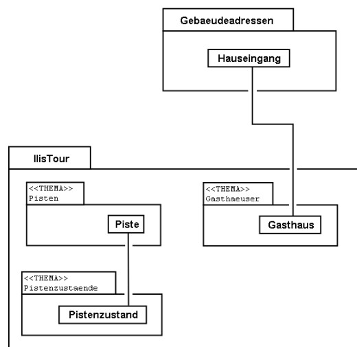
Abbildung 16: Das Ilistaler Tourismus-Modell wird um weitere Themen ergänzt.
