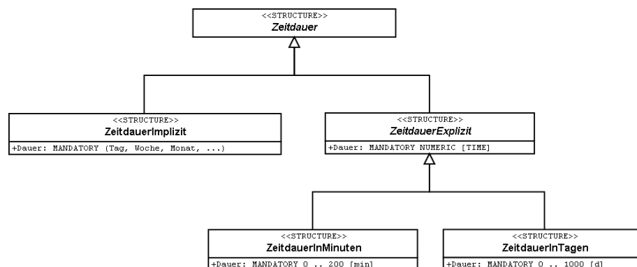
Abbildung 44: Zeitdauer in einer detaillierten Modellierung mit Strukturen. Damit ist es möglich, dass die Gültigkeitsdauer eines Billetts je nach Bedarf ein Monat (ZeitdauerImplizit; links) oder exakt dreissig Tage (ZeitdauerInTagen; rechts) ist.
