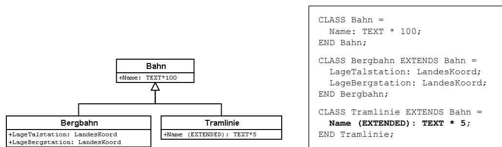
Abbildung 27: Für den Namen einer Tramlinie reichen fünf Zeichen aus: Der Typ der Eigenschaft «Name» wird von der Unterklasse verfeinert (präzisiert). Rechts wiederum dasselbe in der Schreibweise von INTERLIS.
