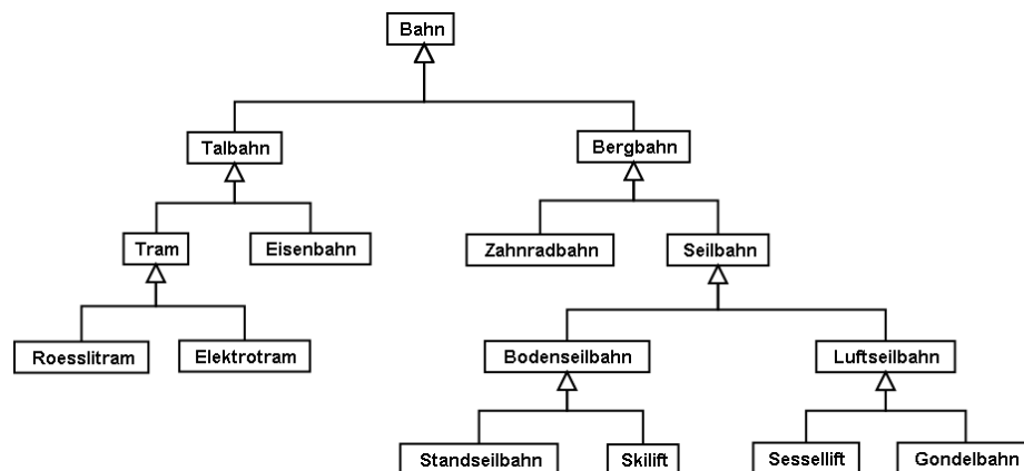
Abbildung 25: Das kraftvolle Mittel der Vererbung kann dazu verleiten, auch dort Spezialfälle zu unterscheiden, wo es von der Anwendung her gar nicht nötig wäre. Zwar ist ein Rösslitrām wirklich nicht ganz dasselbe wie eine elektrische Strassenbahn, aber: Macht es irgendeinen Sinn, all diese Unterscheidungen im Datenmodell zu treffen, oder wird das Ganze so nur unnötig aufgebläht?
