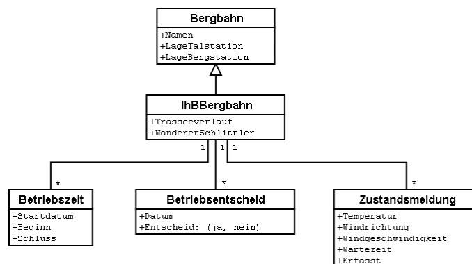
Abbildung 14: Betriebszeiten sind neu als eigenständige Objekte definiert.
