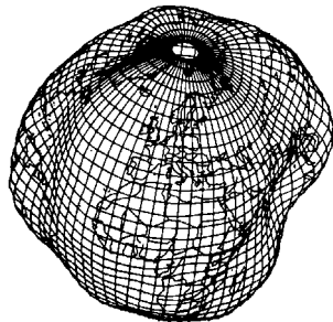
Abbildung 34: Das Schwerefeld der Erde: Beim Geoid wird die Meeresoberfläche in Gedanken unter den Kontinenten fortgesetzt. Gebirgsmassive, Meeresgräben etc. beeinflussen das Schwerefeld und verformen so die gedachte Wasseroberfläche. Diese Zeichnung ist sehr stark überhöht.
