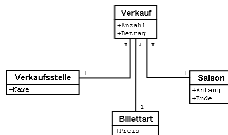
Abbildung 53: Beziehungen zwischen mehr als zwei Beteiligten lassen sich auf gewöhnliche Zweierbeziehungen reduzieren. Die frühere Beziehungsklasse (hier: Verkauf) wird zum gleichberechtigten Partner, und die Beteiligten stehen neu nur noch mit der früheren Beziehungsklasse in Beziehung.
